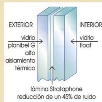
ventanas vidrios laminados tricapa
