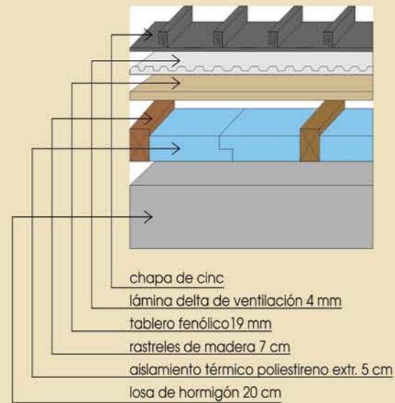
cubierta 5 capas = eficiente aislamiento térmico
