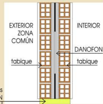
tabiquería interior aislamiento acústico y vibratorio
